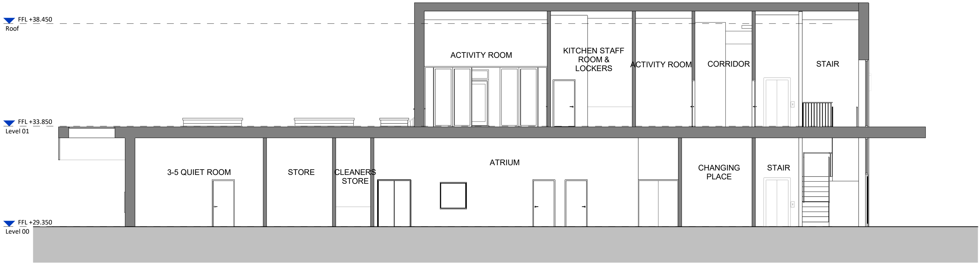
Section A-A 1 : 100
